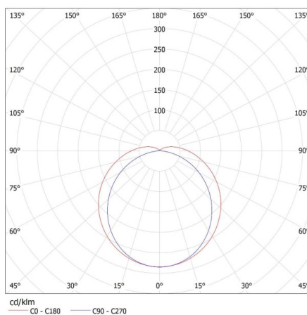
KANLUX S.A. (kat 22603) MAH-LED N 20W-NW / Krzywa rozsyłu światła (biegunowo)
